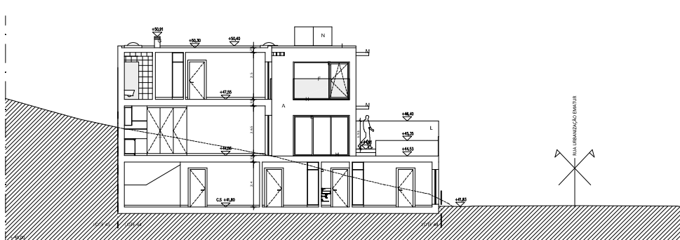
CORTE A
