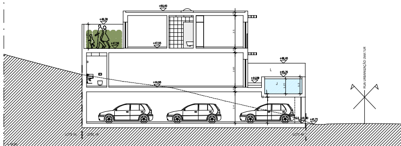
CORTE B
