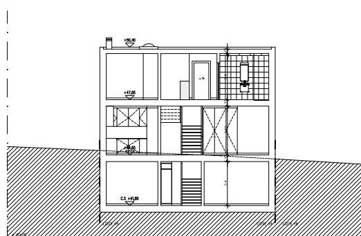
CORTE C
