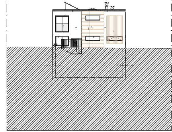
ALÇADO SUL
