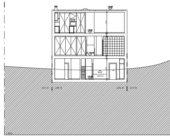
CORTE D
