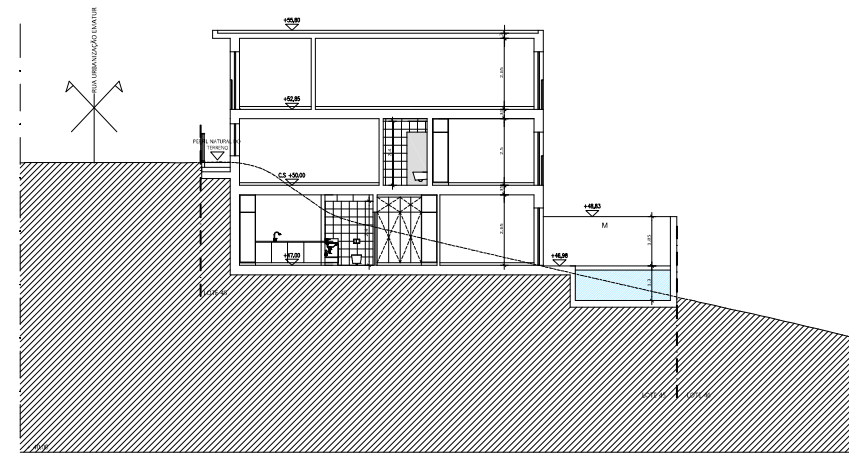
CORTE C
