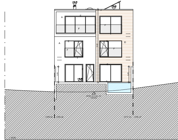
ALÇADO NASCENTE
