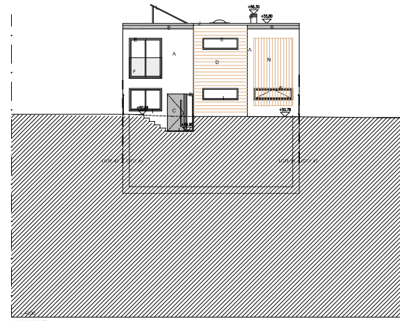
ALÇADO POENTE
