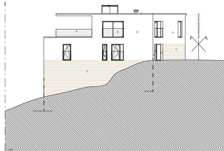
ALÇADO NORTE
