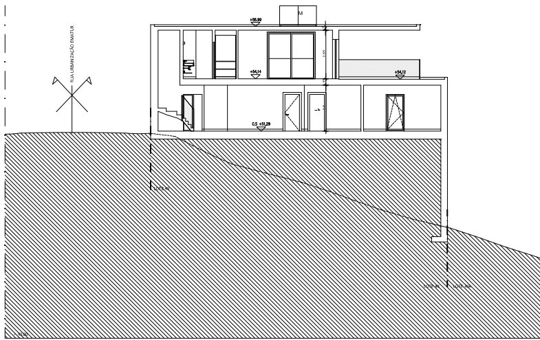
CORTES D
