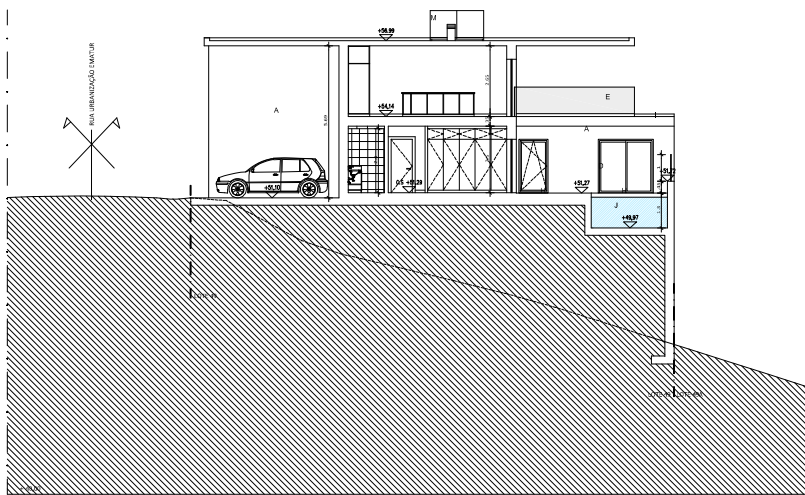
CORTES A
