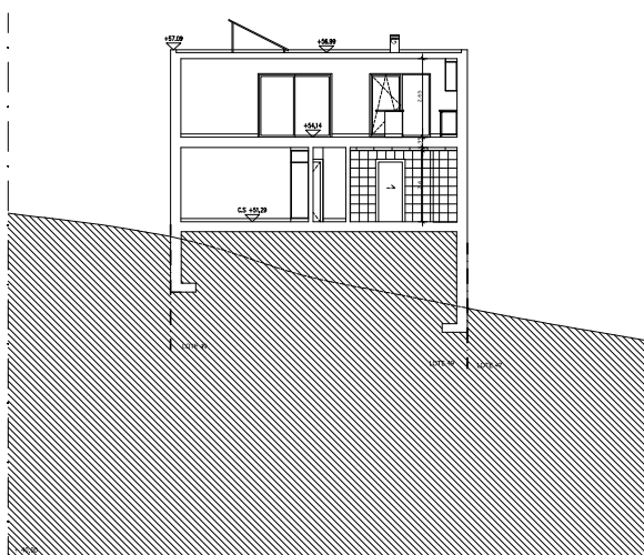
CORTES C
